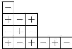
Fig. 1.1. BG-rank
